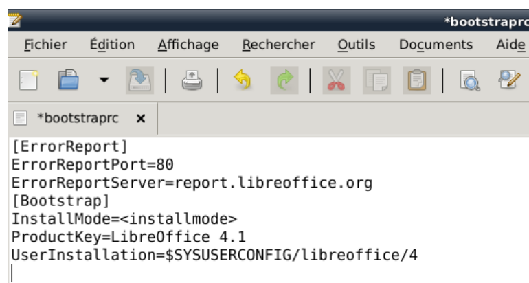
Figure 4 : Le contenu par défaut du fichier d'amorçage
