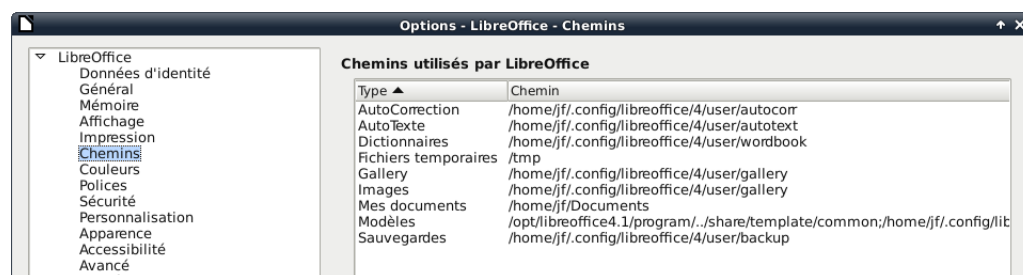
Figure 2 : Les chemins dans LibreOffice. On voit ici (sous Linux), que le profil utilisateur se trouve sous /home/jf/.config/libreoffice/4/user .
